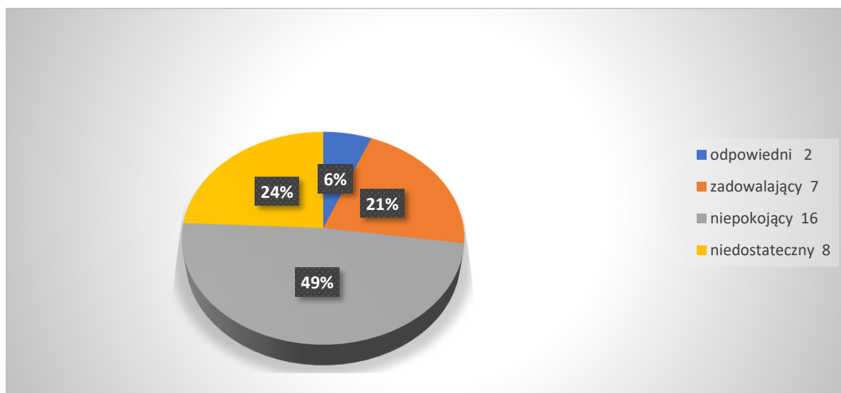
Wykres 7 Podział obiektów mostowych ze względu na ocenę techniczną
